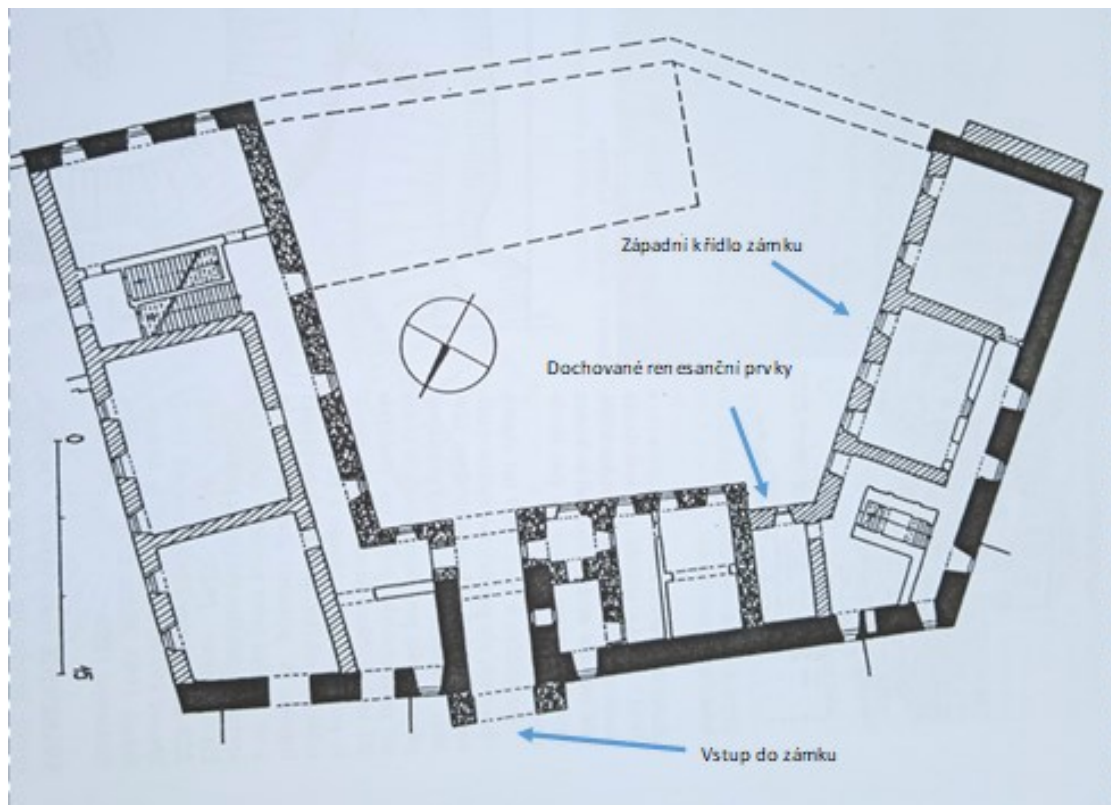
Obrázek 44 Půdorys zámku Šumperk
