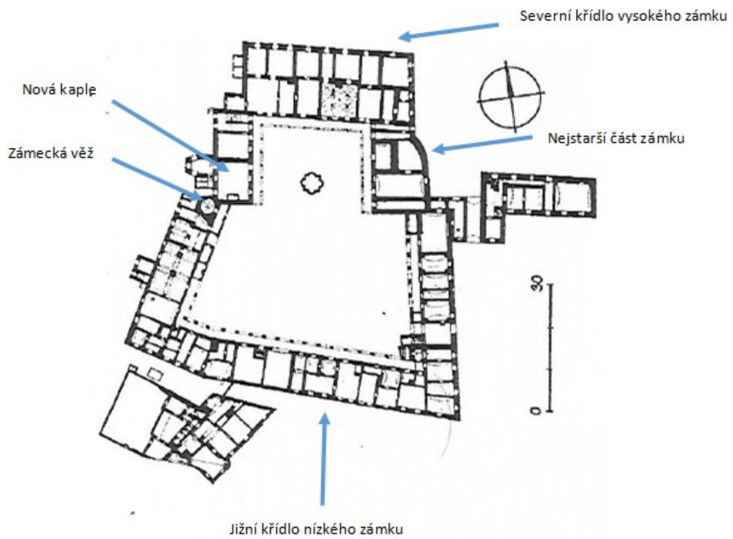
Obrázek 42 Půdorys zámku Velké Losiny
