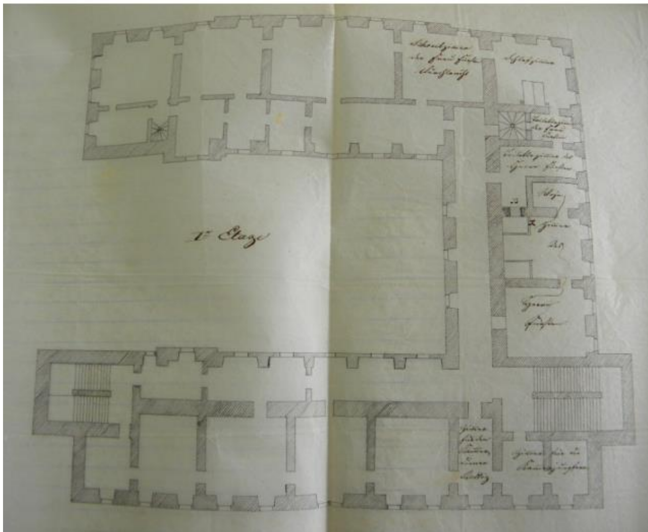
Půdorys první patra chroustovického zámku z 30. let 19. století. 435
