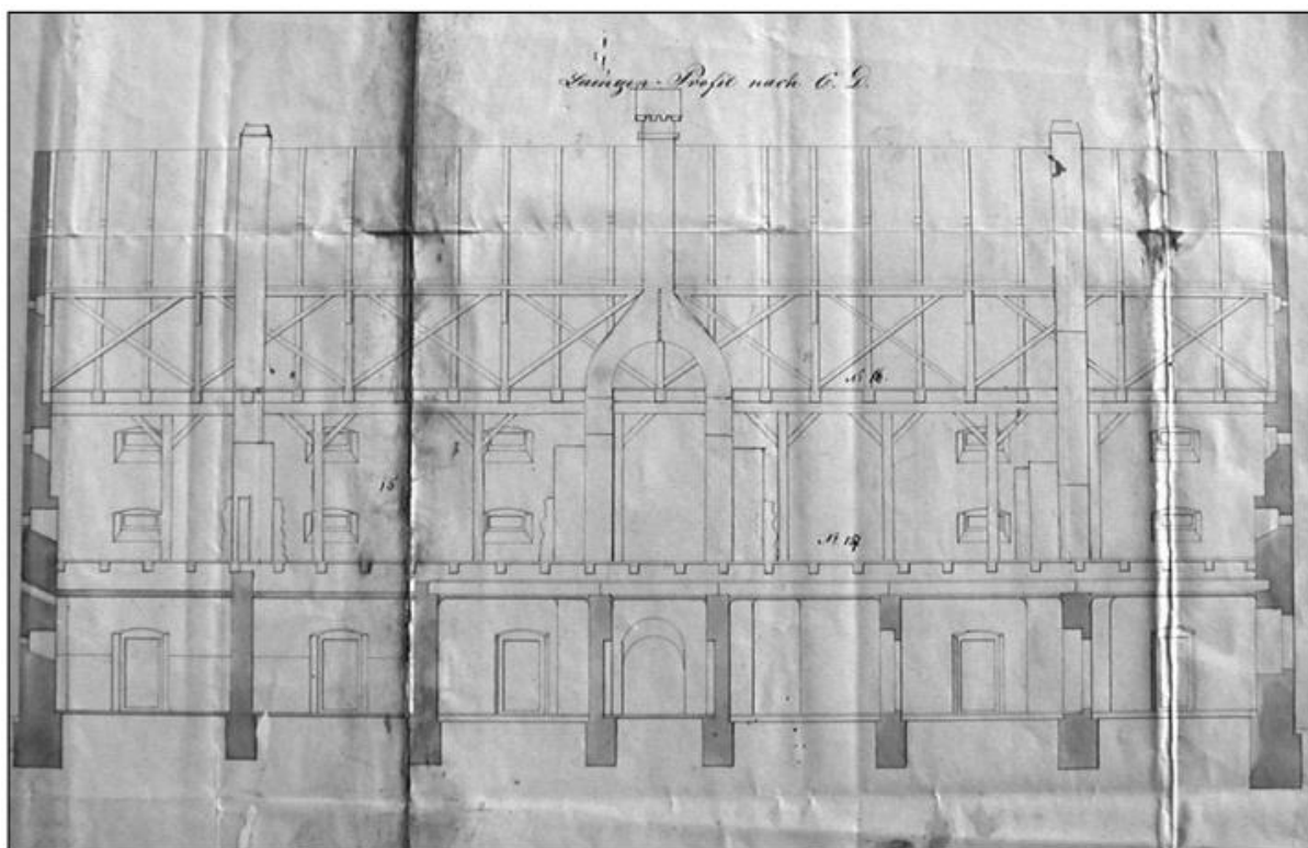
Obr. 7: Čáchnov (okr. Chrudim). Podélný řez stavbou na plánu z roku 1847, který zachycuje horní podlaží jako sýpkové.
