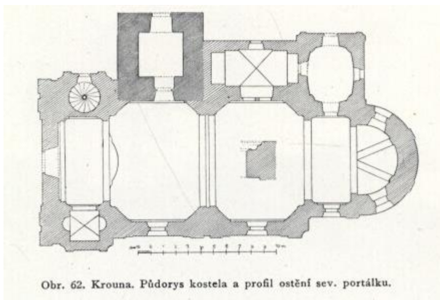
Půdorys kostela sv. Michaela v Krouně 484
