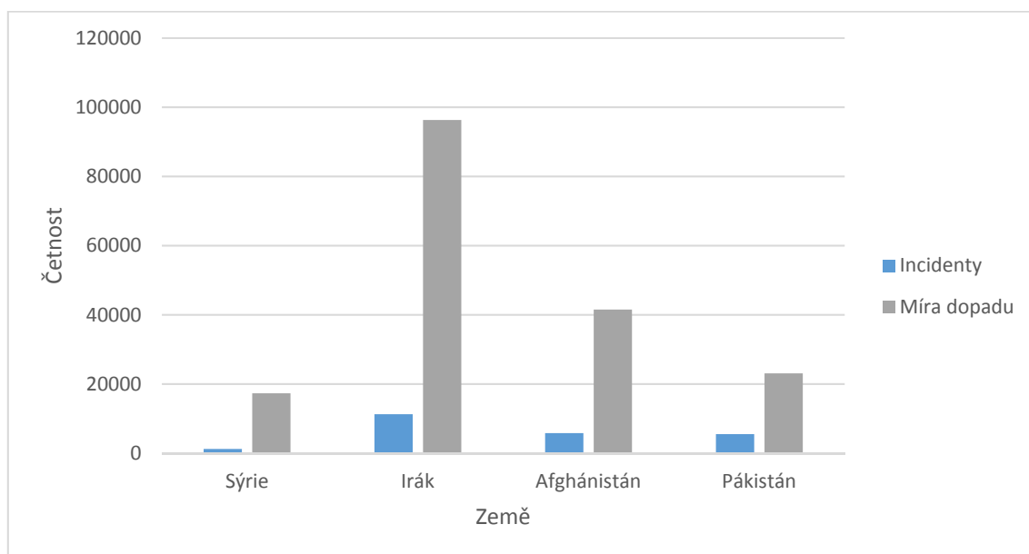
Obrázek 4 - Incidenty a míra dopadu (Sýrie, Irák, Afghánistán, Pákistán)
