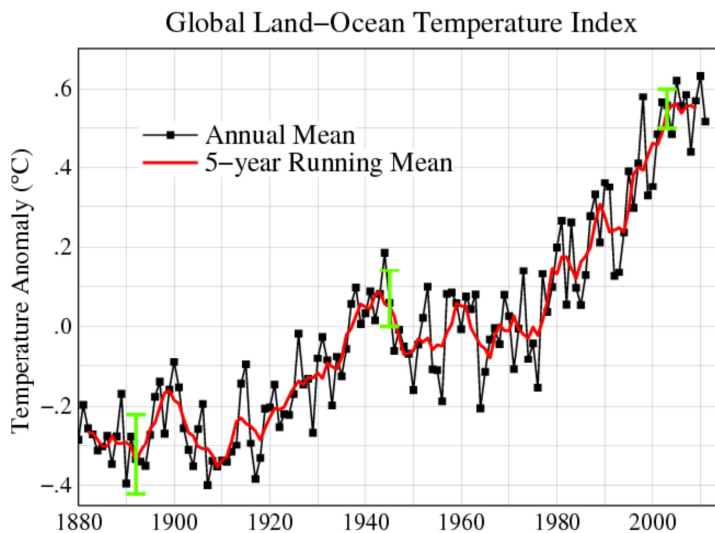
Graf 3. 1 Vývoj globálního teplotního indexu
