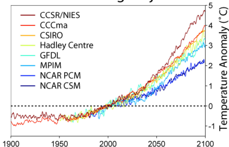
Graf 3. 5 Scénáře vývoje klimatu v budoucnosti
