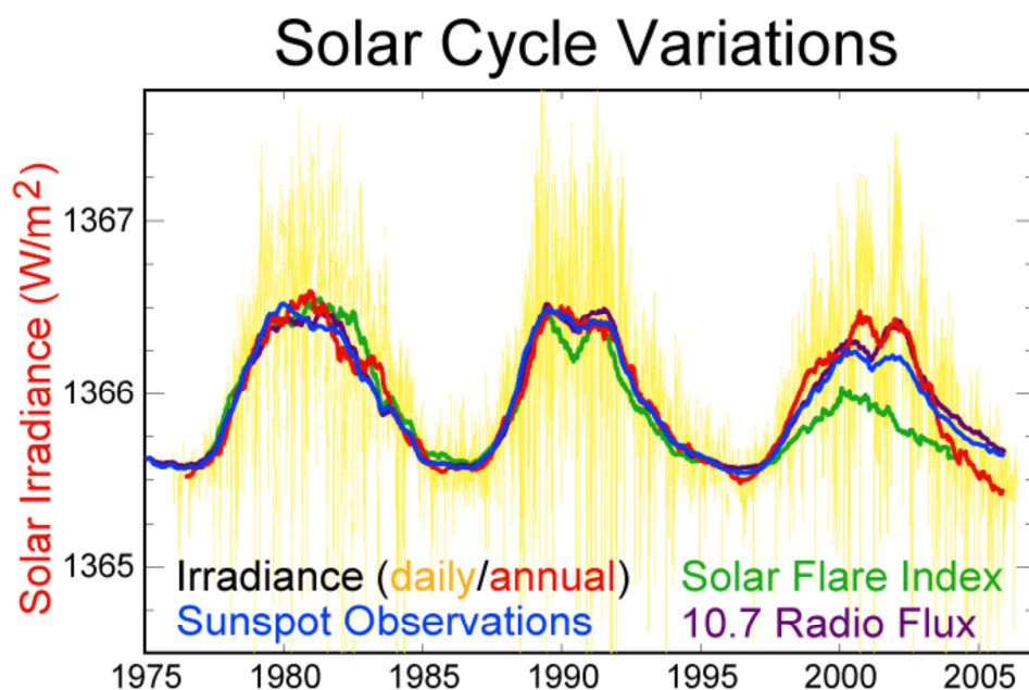
Graf 3.3 Solární cyklus
