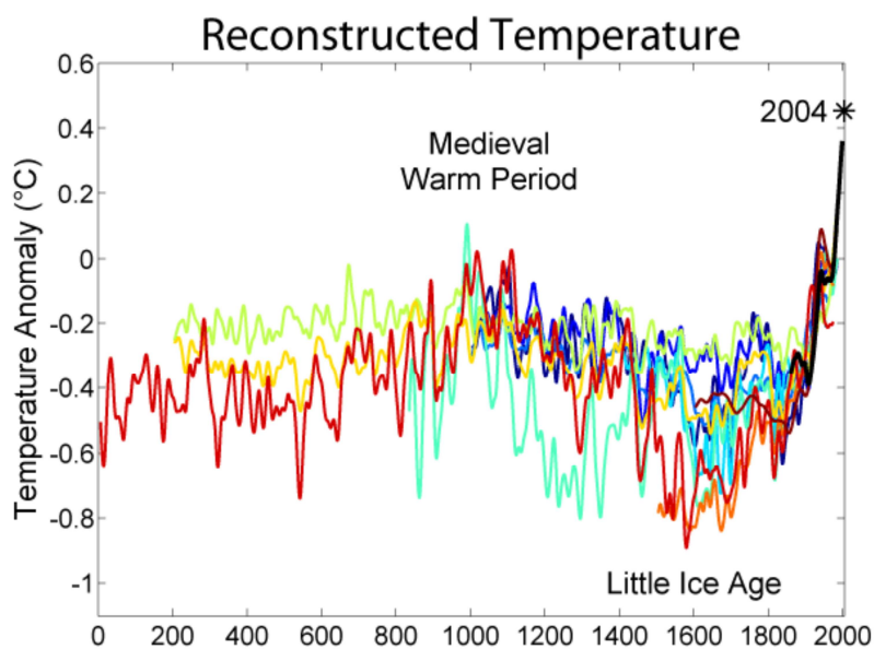
Graf 3. 2 Rekonstrukce vývoje teploty
