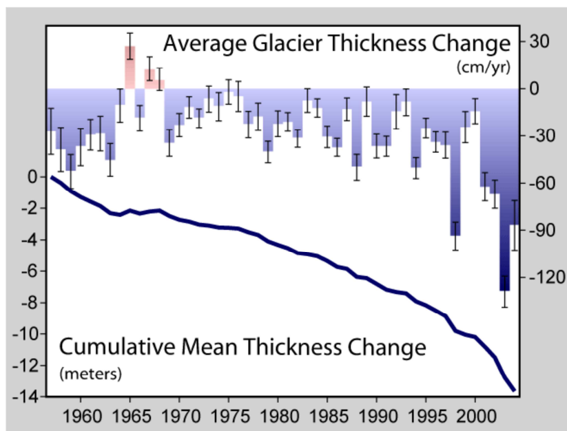
Graf 3.4 Vývoj poklesu tloušťky ledovců
