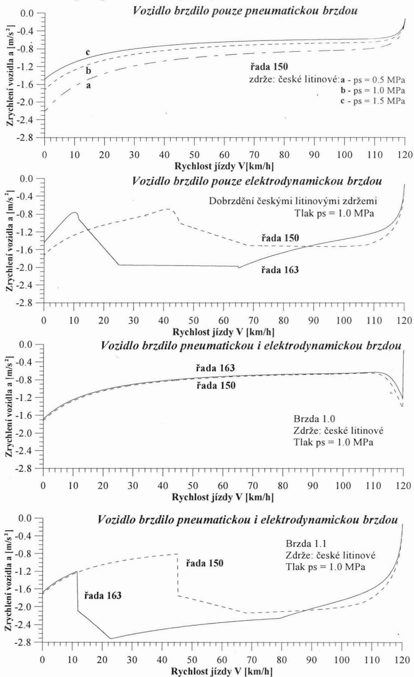
Obr. 5 Závislost zrychlení vozidla a na rychlosti jízdy V
