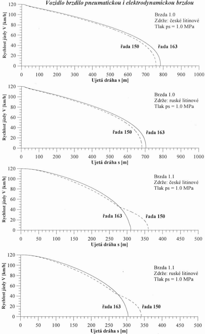
Obr. 4 Závislost poklesu rychlosti V na ujeté dráze s
