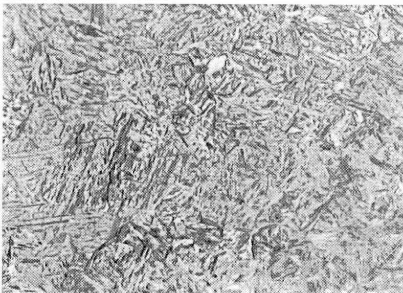
Obr. 1 Mikrostruktura lité oceli Lo8CrNiMo, zv. 100 x
