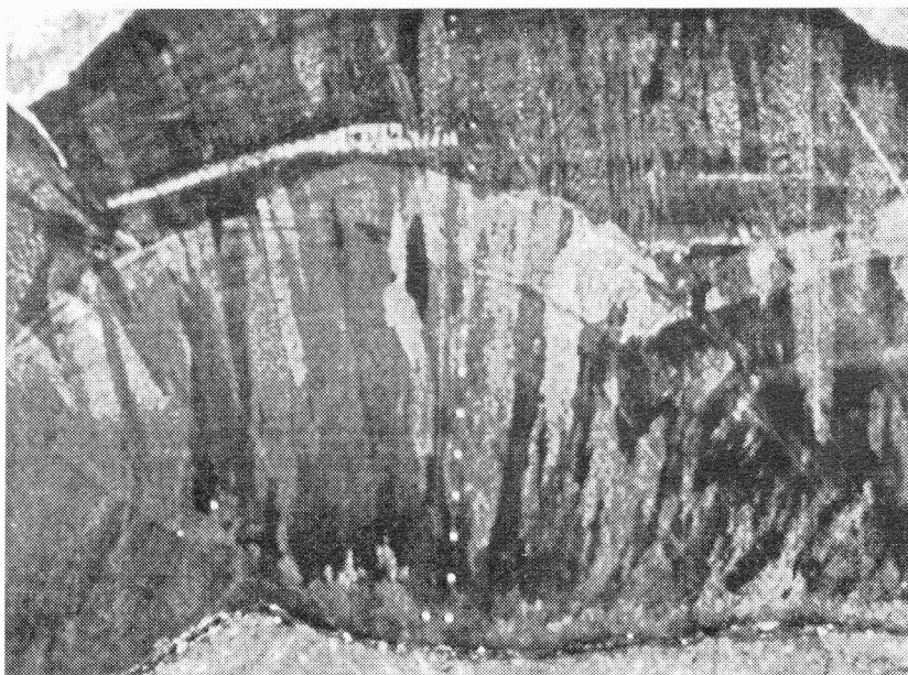
Obr. 4 Dendritická stavba austenitických návarů, zv. 63 x
