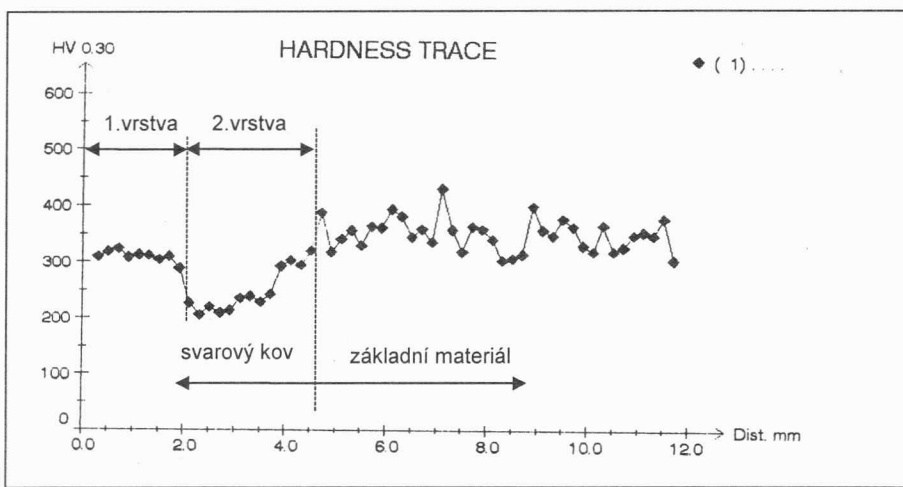
Obr. 6 Průběh mikrotvrdosti [HVm] pro „tvrdočávar“
