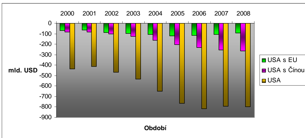
Graf 5-21: Obchodní bilance USA, obchodní bilance USA s EU a obchodní bilance USA s Čínou
